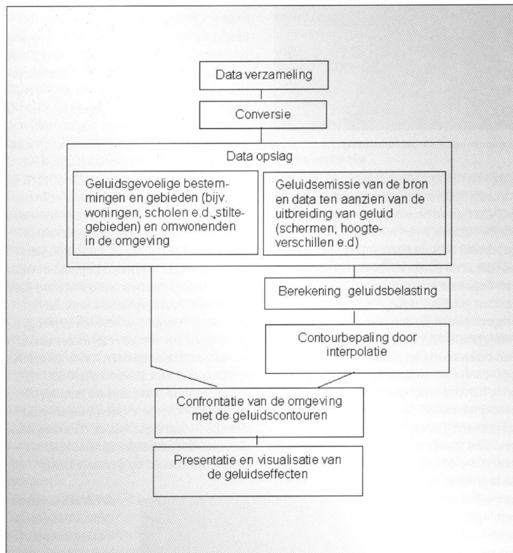
Figuur 1: schematisatie van het noise-mapping proces.
