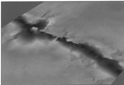
Figuur 3: continu beeld van de geluidsbelastingen na interpolatie op basis van de rekenpunten.
