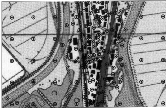
Figuur 2: dichtheid van rekenpunten afhankelijk van de te verwachten variatie in geluidsbelasting.
