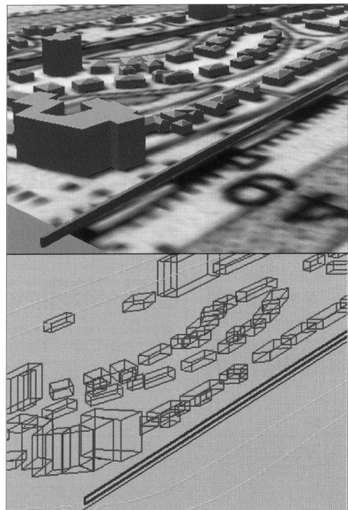
Figuur 5: genereren van een akoestisch model uit topografische ondergronden en 3-D informatie.
