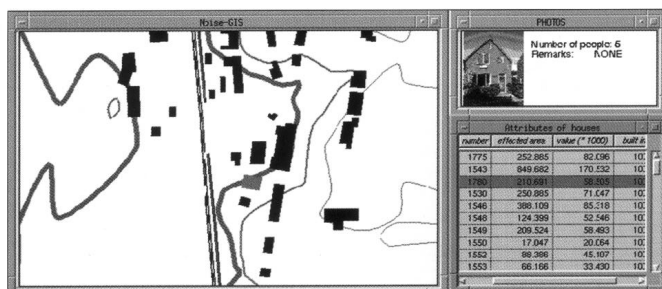
Figuur 4: bepaling van het aantal geluidsbelaste woningen door combinatie van de geluidsc contouren en de nabijgelegen woningen.
